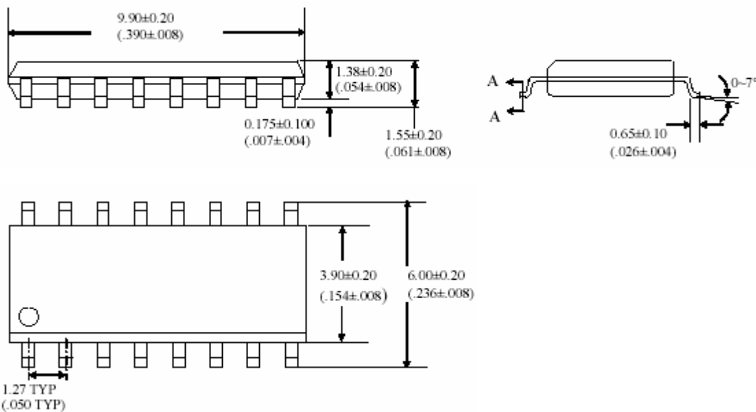
SOP16L
